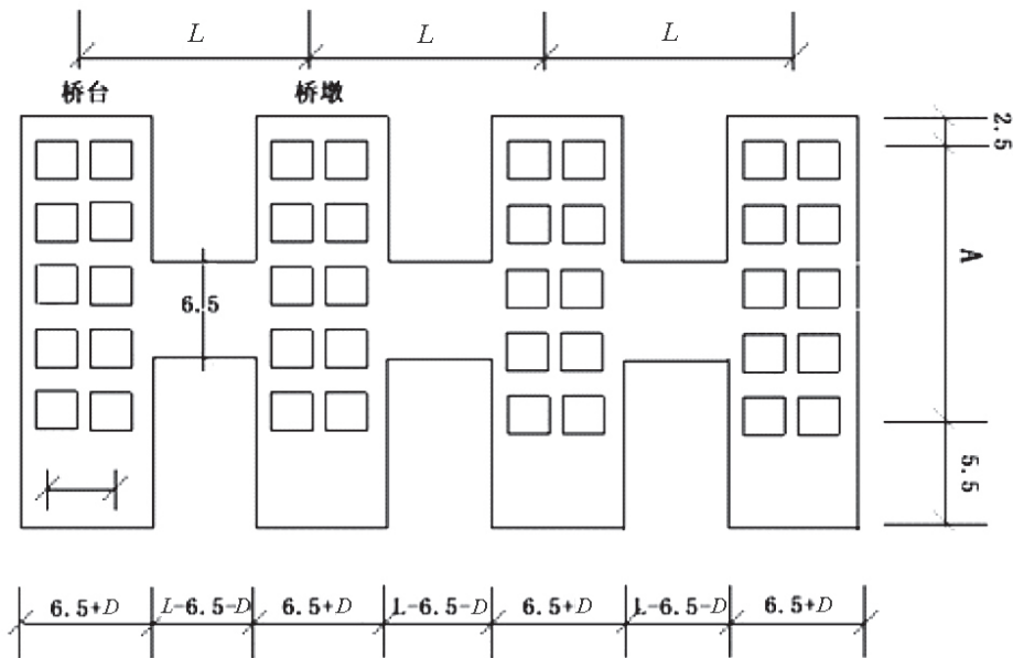
工作平台面积计算示意图
