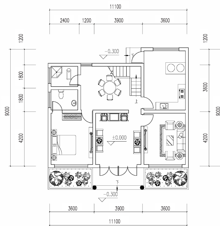
一层平面图
