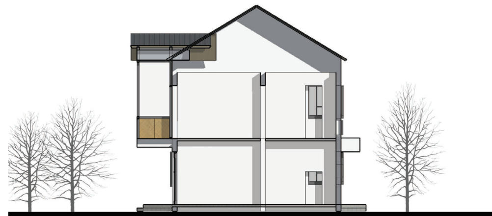
1-1 剖面图
