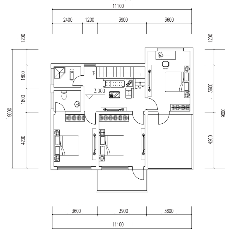
二层平面图
