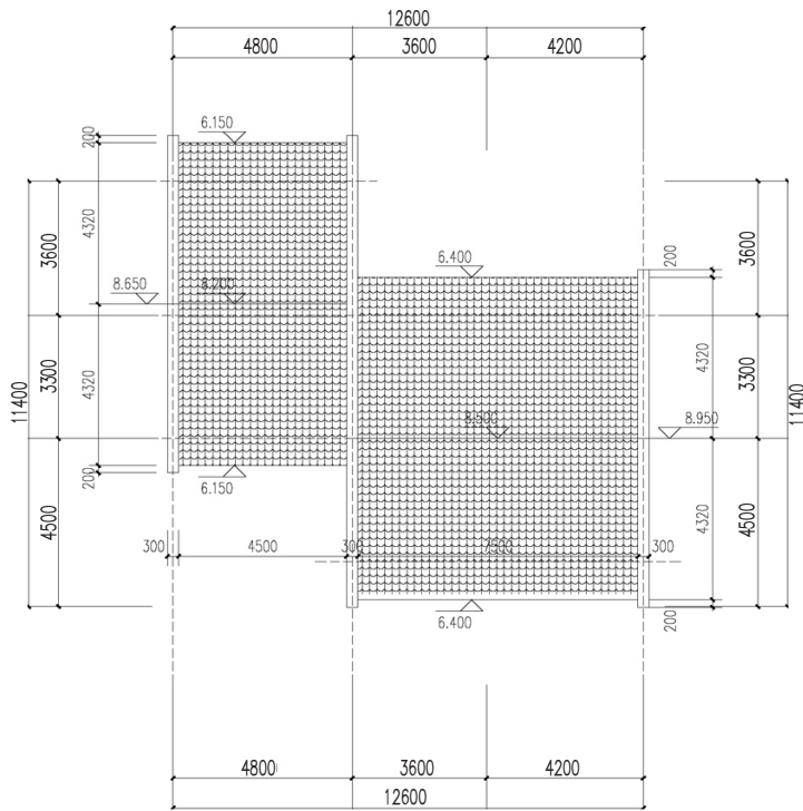
屋顶平面图
