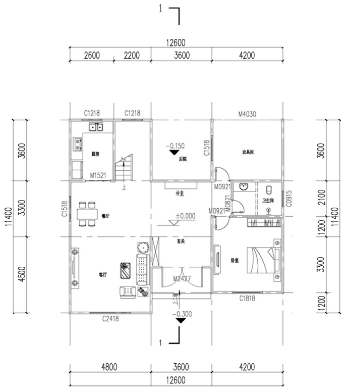
一层平面图
