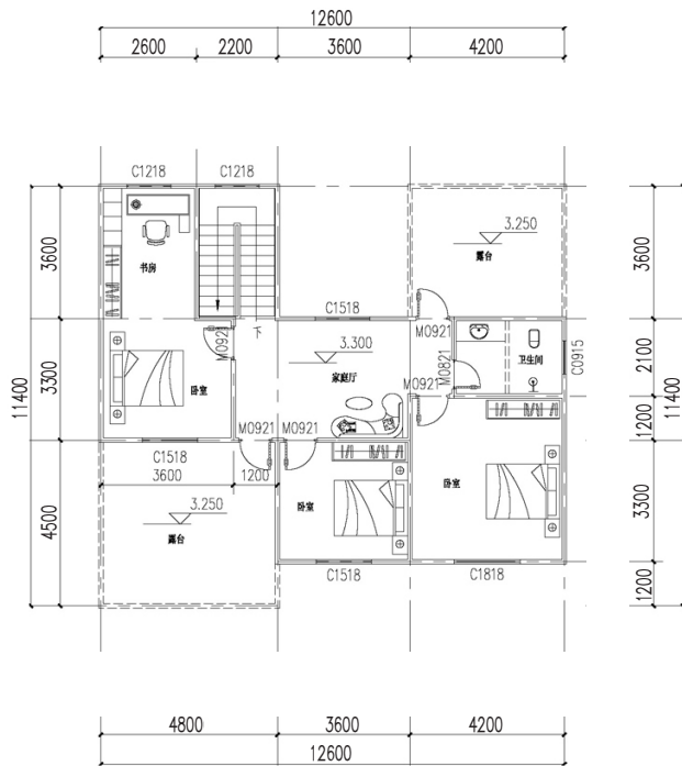
二层平面图
