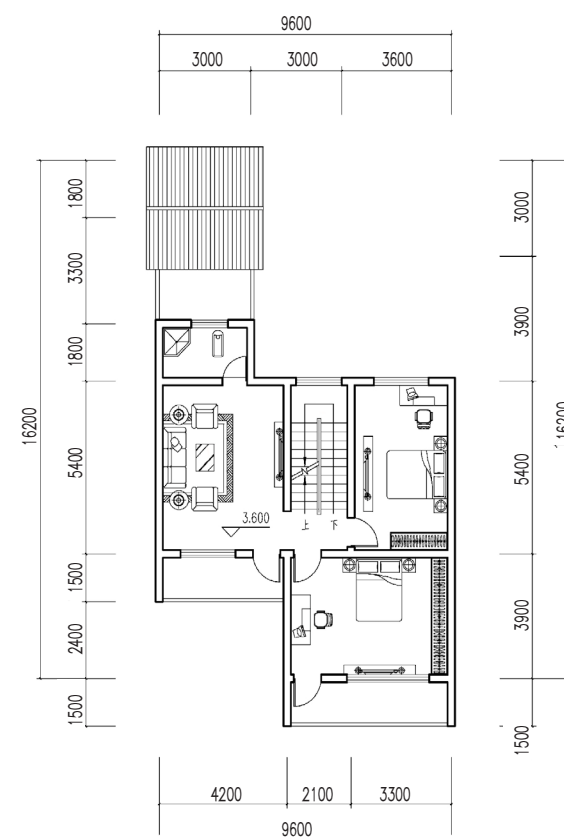
二层平面图
