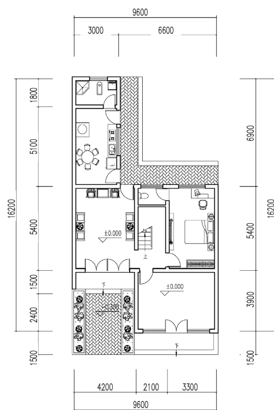
一层平面图
