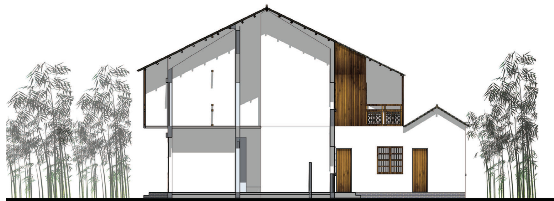
1-1 剖面图
