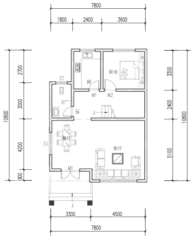
一层平面图
