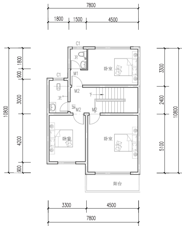
二层平面图
