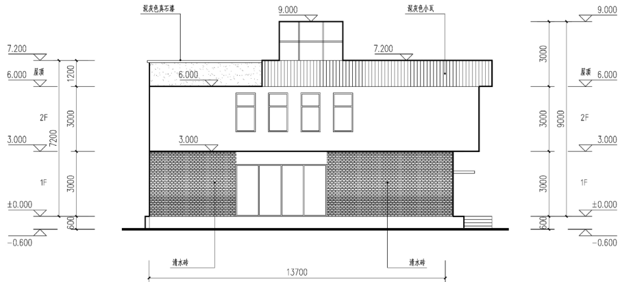
西立面图
