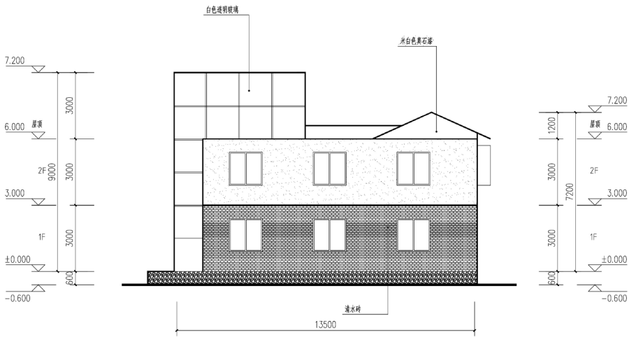
北立面图
