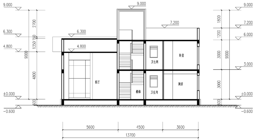
剖面图
