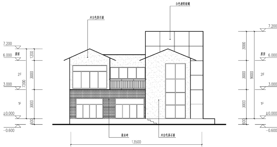
南立面图
