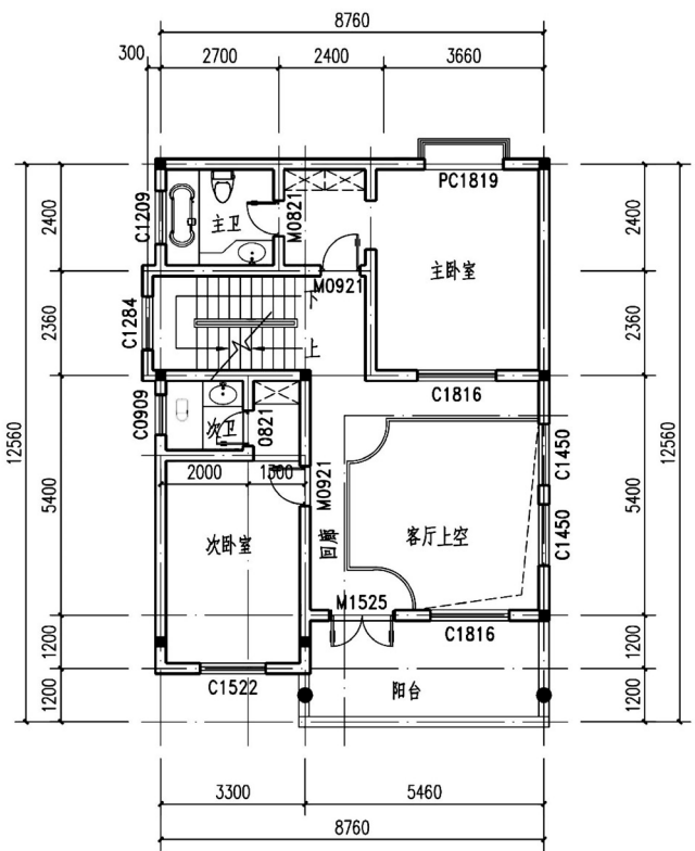
二层平面图
