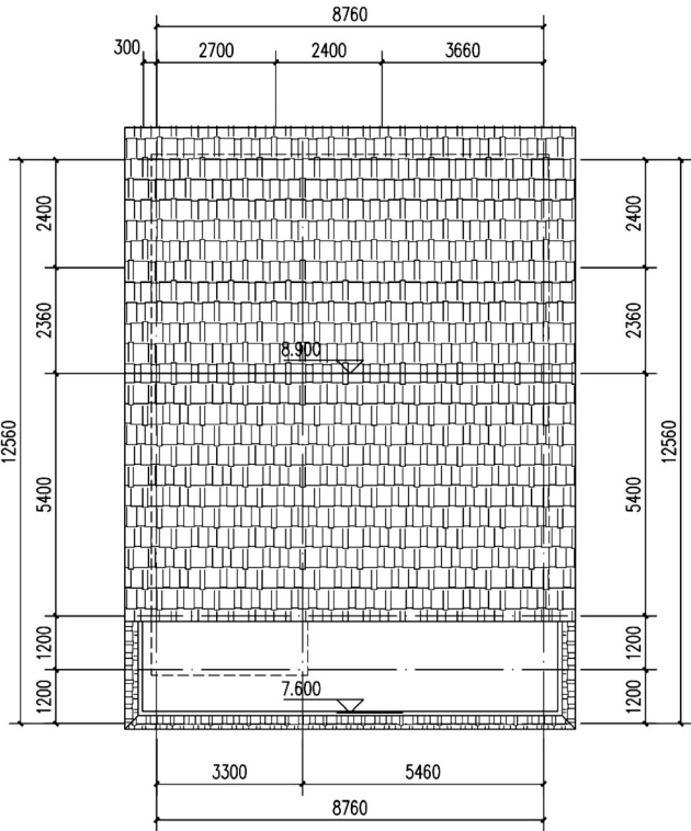
屋顶平面图
