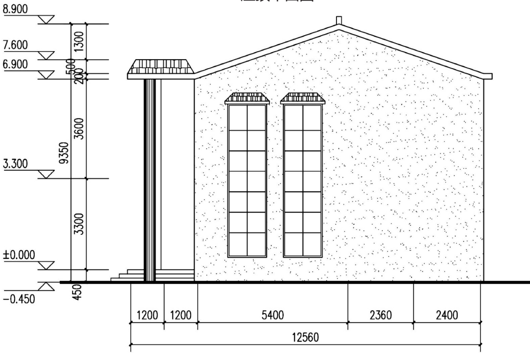
侧立面图
