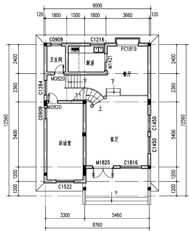
一层平面图
