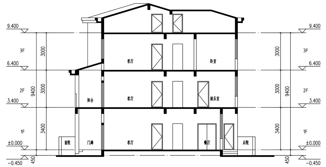
剖面图
