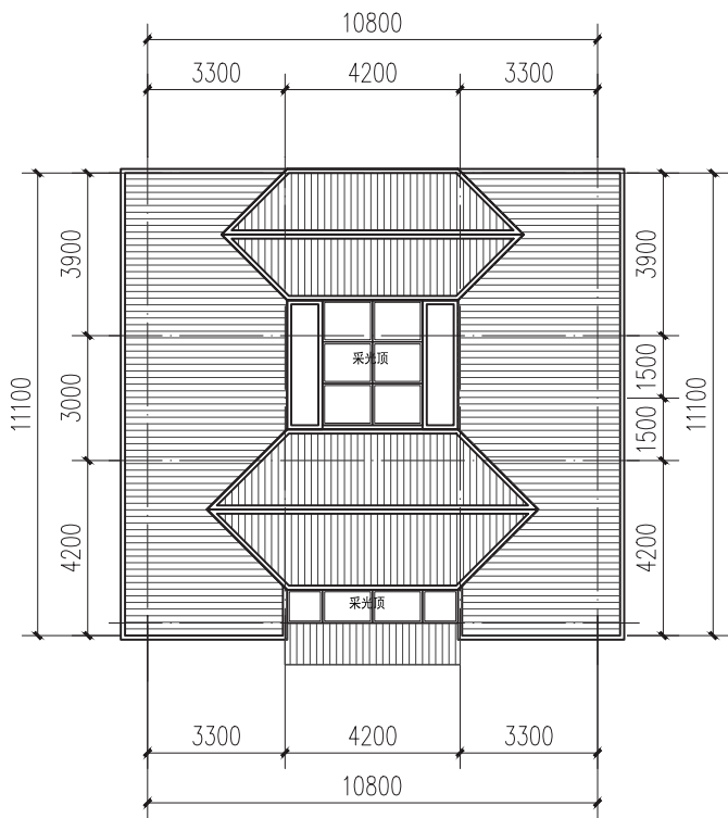
屋顶平面图
