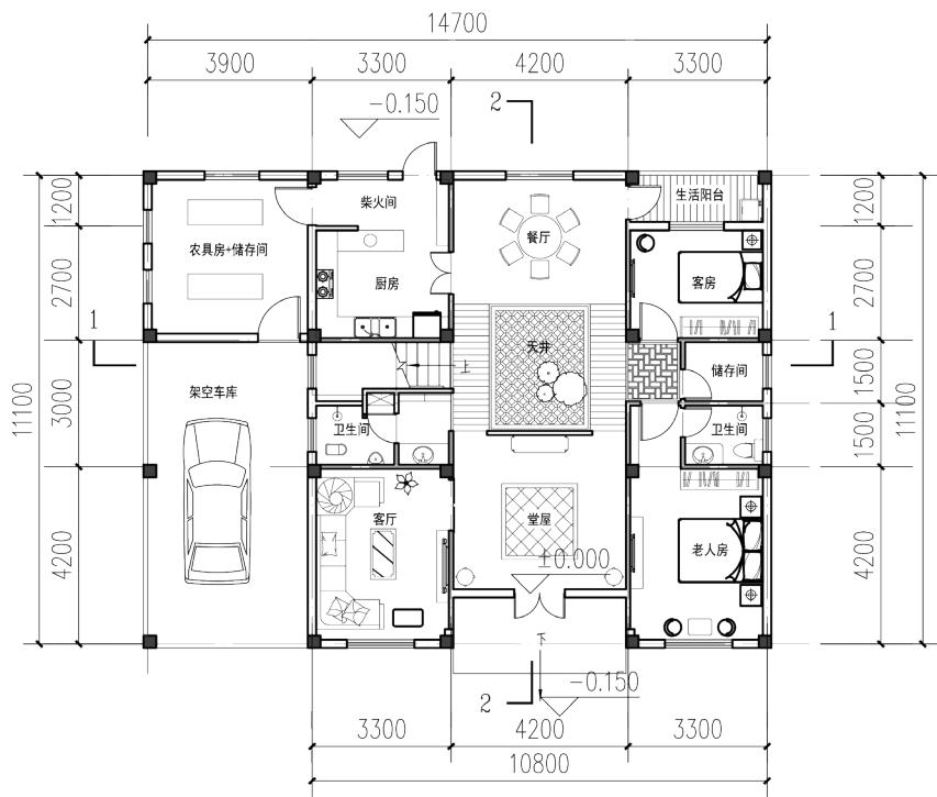
一层平面图
