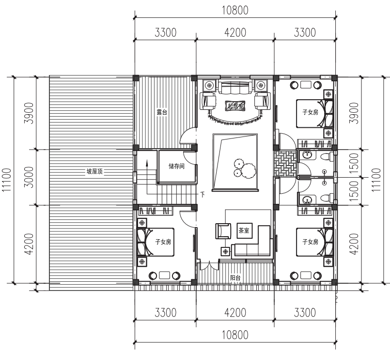
二层平面图
